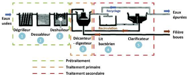
Succession des étapes d'assainissement des eaux usées par le système de lit bactérien
